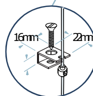
Squadretta / Parete
