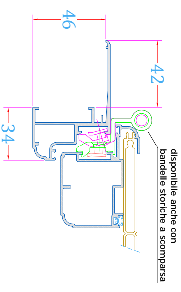
MIXER SCURONE su TELAIO INSINUA aletta 42 mm e cerniere a camera europea
