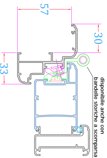
FLORENTIA STORICA su TELAIO INSINUA aletta 30 mm e cerniere a camera europea
