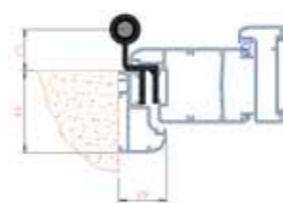
INSINUA FLORENTIA con telaio rifilato in ELLE. Bandelle storiche.
