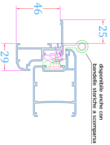
MIXER STORICA su TELAIO INSINUA aletta 25 mm e cerniere a camera europea
