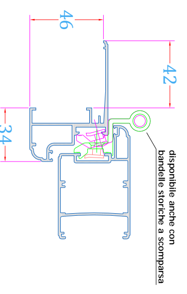
MIXER STORICA su TELAIO INSINUA aletta 42 mm e cerniere a camera europea
