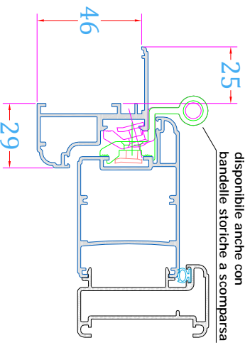
FLORENTIA STORICA su TELAIO INSINUA aletta 25 mm e cerniere a camera europea
