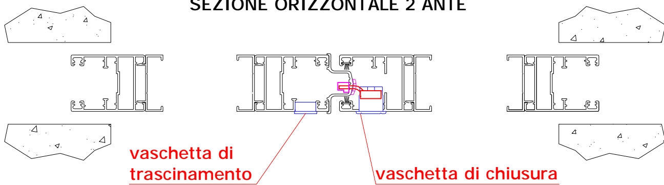
SEZIONE ORIZZONTALE 2 ANTE
